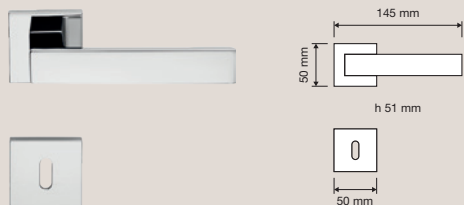
505 RB 024 Maniglia con rosetta ribassata art.024 / Door handle on reduced rose art.024
