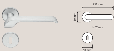
470 RB 027 Maniglia con rosetta art.027 / Door handle on rose art.027
