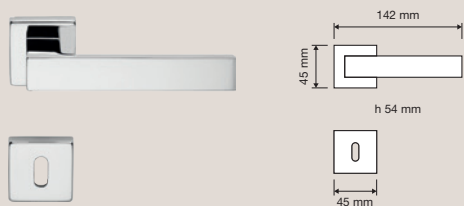
505 RB 014 Maniglia con rosetta art.014 / Door handle on rose art.014
