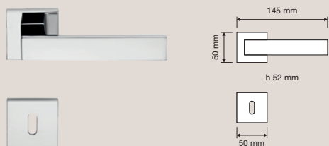
505 RB 088 Maniglia con rosetta art.088 / Door handle on rose art.088
