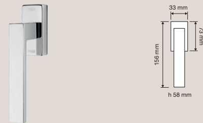
505 SK Maniglia per finestra con movimento DK SmartBlock / Window handle with DK SmartBlock movement
