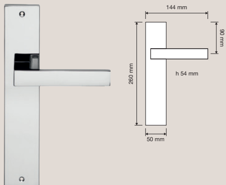
475 PL Maniglia con placca art.475 / Door handle on plate art.475
